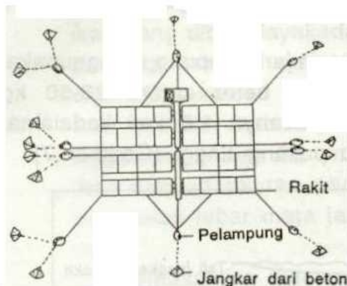
Gambar 8. Rancangan Tata Letak Kerangka Kurungan Jaring Apung
