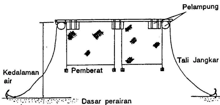
Gambar 4. Disain Konstruksi Kurungan Apung
