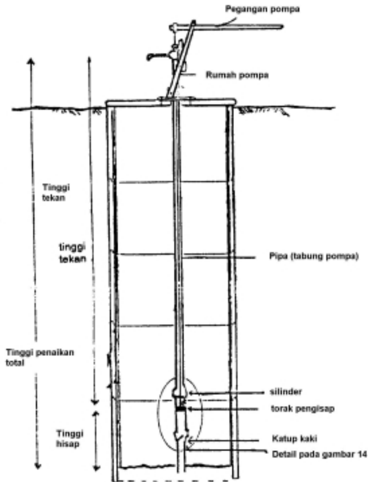
Gambar 13. Suku Cadang Utama Sebuah Pompa Hisap
